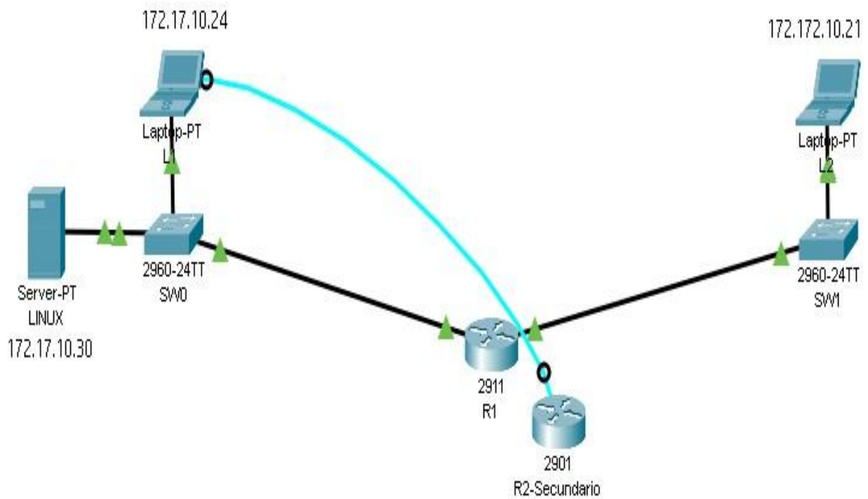
Figura1. Posible RED LAN Conexión de 2 Centros Universitarios
